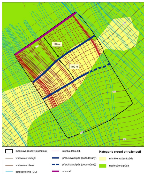
Obr. 2-45: Souvrat' S3 na spodní hranici DPB doplněna o přerušovací pás ve vzdálenosti do 200 m od horní hrany souvratě proti směru odtokových linií, protože vzdálenost od horní hrany prvního přerušovacího pásu proti směru odtokových linií k horní hranici plochy MEO je větší než 200 m. Další přerušovací pás není nutné aplikovat, protože vzdálenost od horní hrany druhého přerušovacího pásu proti směru odtokových linií k horní hranici plochy MEO je menší než 200 m. (přerušovaně zobrazeno doporučené opatření)
