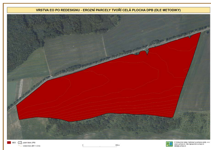
Obr. 2-6: Vrstva EO po redesignu – erozní parcely tvoří celá plocha DPB
