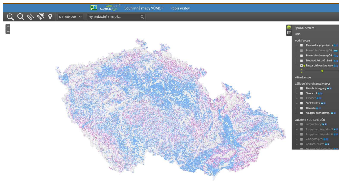
Obr. 7-8: Souhrnné mapy VÚMOP
