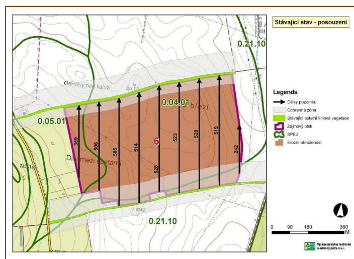
Obr. 6-12: Ukázkový díl půdního bloku s vyznačeným převládajícím směrem větru a stanovenou maximální délkou pozemku (černé šipky s uvedením délky)
