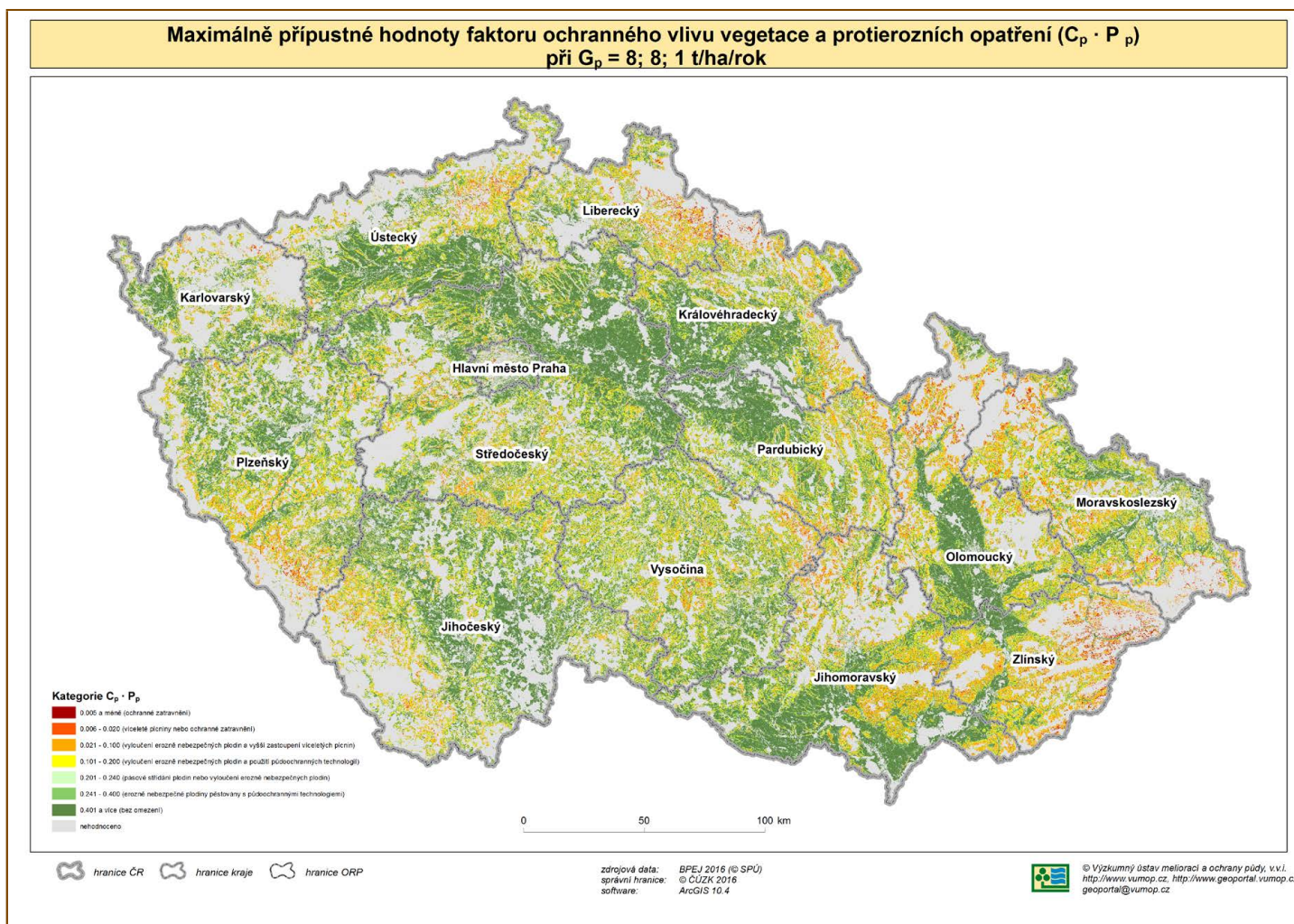
Obr. 3-7: Mapa Maximální přípustné hodnoty faktoru ochranného vlivu vegetace a protierozních opatření ( C_p \cdot P_p )
