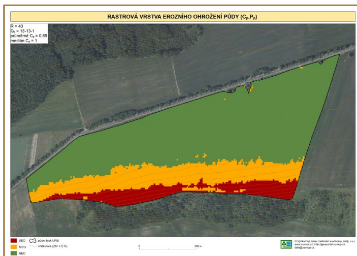
Obr. 2-9: Rastrová vrstva erozního ohrožení půdy ( C_p \cdot P_p )
