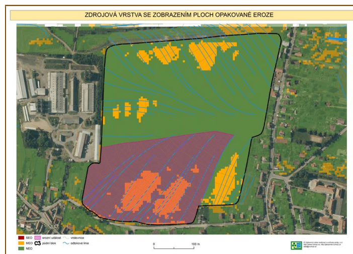
Obr. 2-24: Vymezení erozně uzavřeného celku (EUC) pro přehrazení
