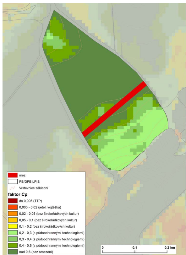
Obr. 2-18: Mapa Maximálních přípustných hodnot faktoru ochranného vlivu vegetace a faktoru protierozních opatření C_p \cdot P_p na DPB s implementovaným krajinným prvkem
