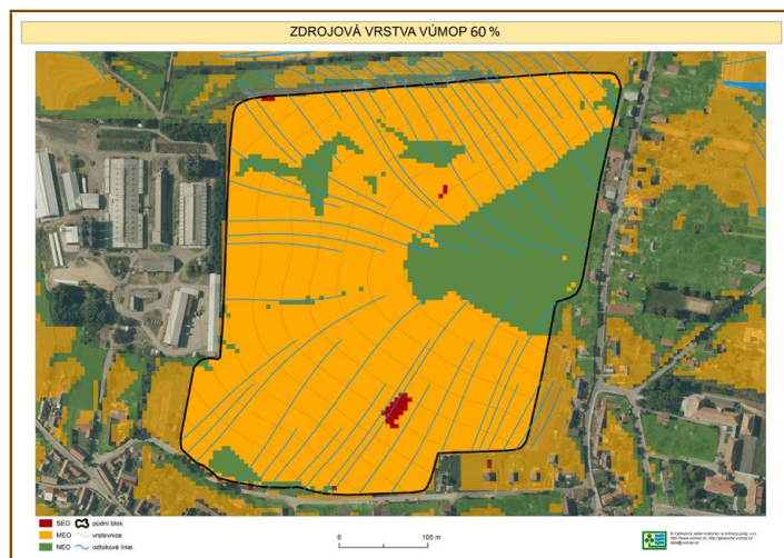
Obr. 2-23: Nová podkladová rastrová vrstva EO od 1. I. 2030
