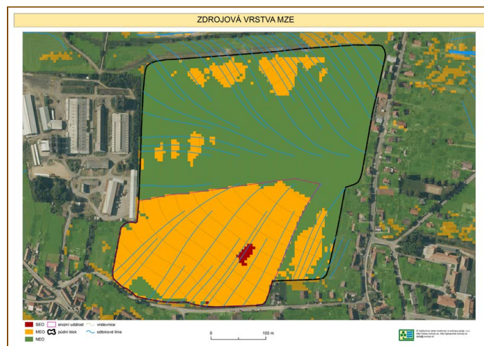
Obr. 2-25: Nová podkladová rastrová vrstva EO po zpřísnění na daném EUC
