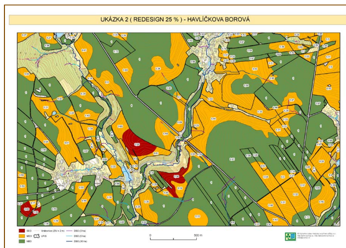
Obr. 2-5: Vrstva EO přepočítaná na erozní parcely, čísla uvedená u erozních parcel představují mediánovou hodnotu C_p \cdot P_p
