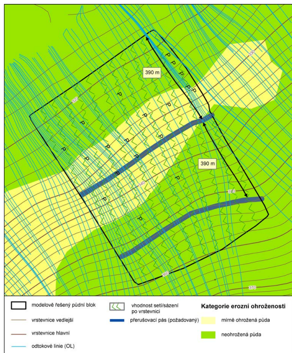
Obr. 2-48: Setísázení po vrstevnici doplněno přerušovacím pásem na DPB s průměrnou sklonitostí nad 5°
