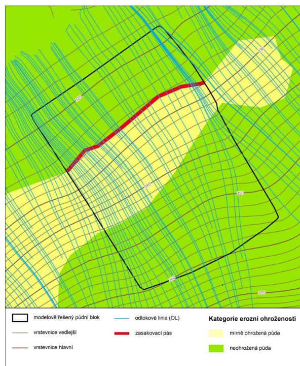
Obr. 2-33: Zasakovací pás založen na spodní hranici plochy MEO
