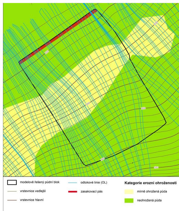
Obr. 2-32: Zasakovací pás založen na spodní hranici DPB
