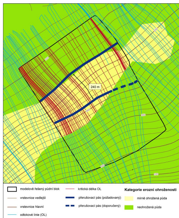
Obr. 2-30: Přerušovací pásy na PB/DPB se sklonitostí 3–5° (přerušované zobrazeno doporučené opatření)
