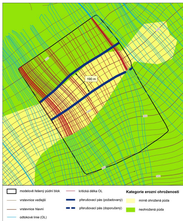
Obr. 2-31: Přerušovací pásy na DPB se sklonitostí nad 5° (přerušované zobrazeno doporučené opatření)
