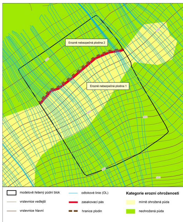
Obr. 2-34: Zasakovací pás založen na spodní hranici souvislé plochy plodiny zasahující do plochy MEO
