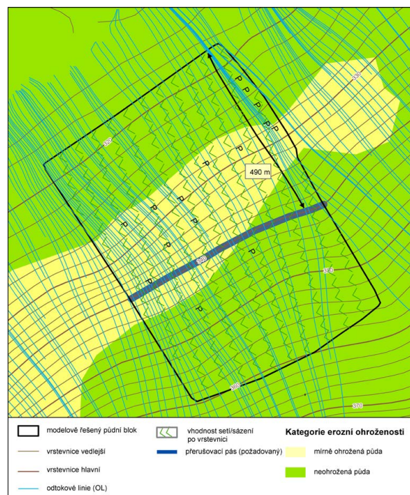
Obr. 2-47: Setí/sázení po vrstevnici doplněno přerušovacím pásem na DPB s průměrnou sklonitostí 3–5°
