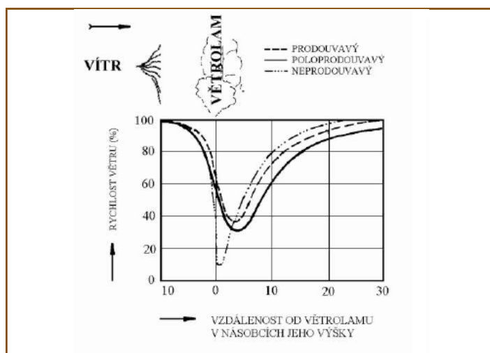
Obr. 6-9: Schéma účinnosti různých typů větrolamů
