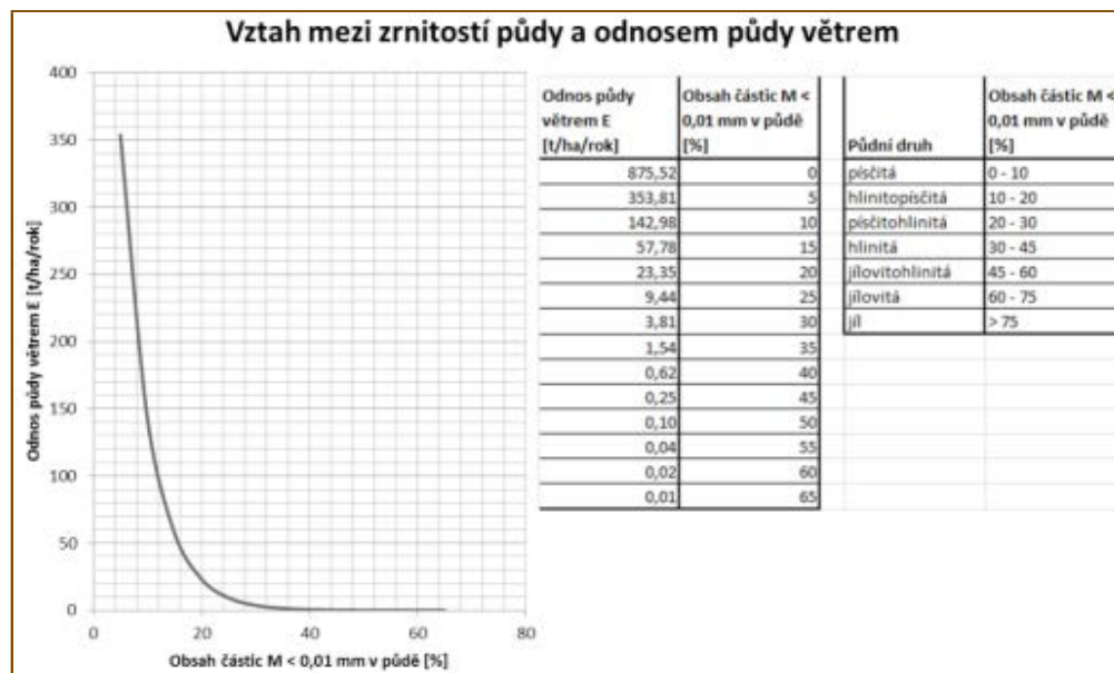
Obr. 6-11: Nomogram pro odhad erodovatelnosti půdy větrem podle Pasáka a kol. (1984)
