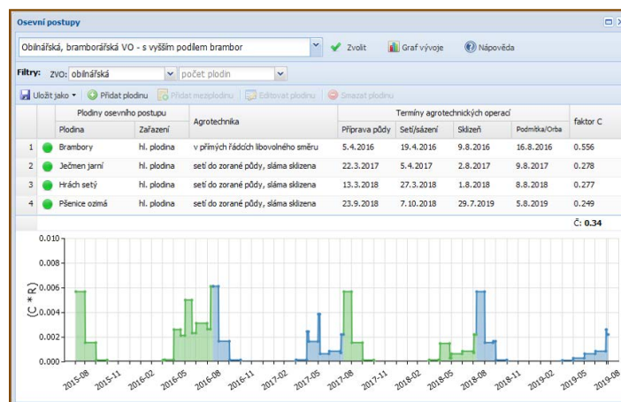
Obr. 2-10: Vyhodnocení ochranného účinku osevního postupu v Protierozní kalkulačce
