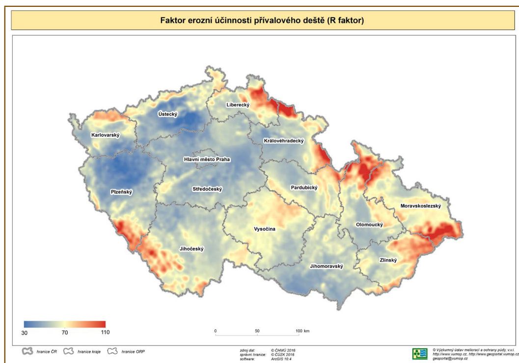
Obr. 2-21: Mapa faktoru erozní účinnosti deště R
