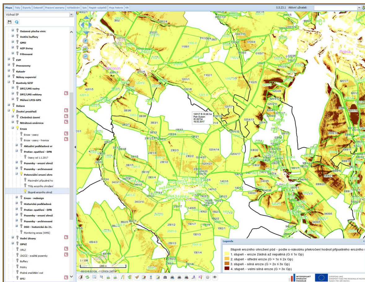
Obr. 7-5: Stupně erozní ohroženosti; zobrazení v LPIS
