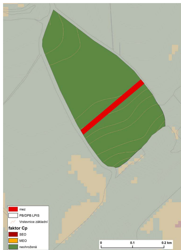
Obr. 2-19: Vrstva erozní ohroženosti v rámci Standardu DZES 5 na DPB s implementovaným krajinným prvkem
