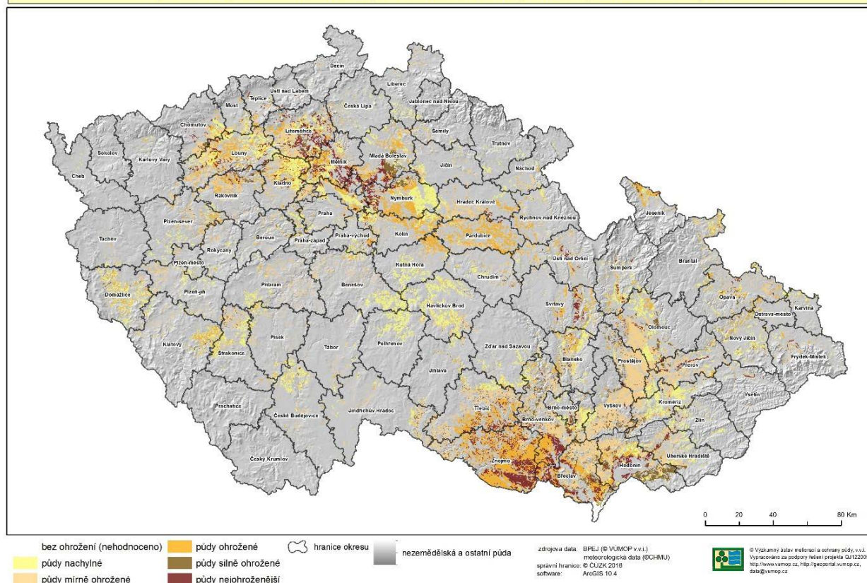
Obr. 6-14: Mapa oblastí potenciálně ohrožených větrnou erozí na podkladu půdně-klimatických faktorů
