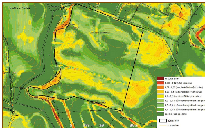
Obr. 3-9: Ohroženost půdy vodní erozí podle C_p \cdot P_p
