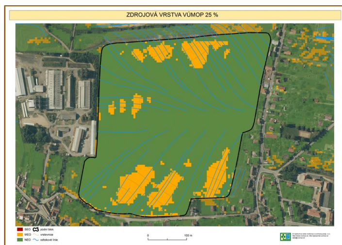
Obr. 2-22: Nová podkladová rastrová vrstva EO od 1. I. 2018
