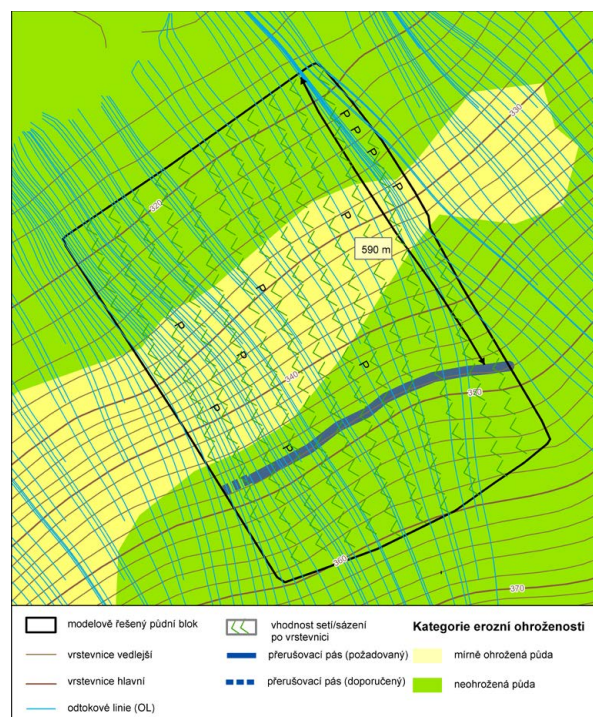
Obr. 2-46: Setí/sázení po vrstevnici doplněno přerušovacím pásem na DPB s průměrnou sklonitostí do 3° (přerušovaně zobrazeno doporučené opatření)
