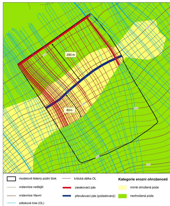
Obr. 2-36: Zasakovací pás Z1 založen na spodní hranici DPB doplněn o přerušovací pás ve vzdálenosti do 300 m od horní hrany zasakovacího pásu proti směru odtokových linií. Další přerušovací pás není nutné aplikovat, protože vzdálenost od horní hrany prvního přerušovacího pásu proti směru odtokových linií k horní hranici plochy MEO je menší než 300 m.
