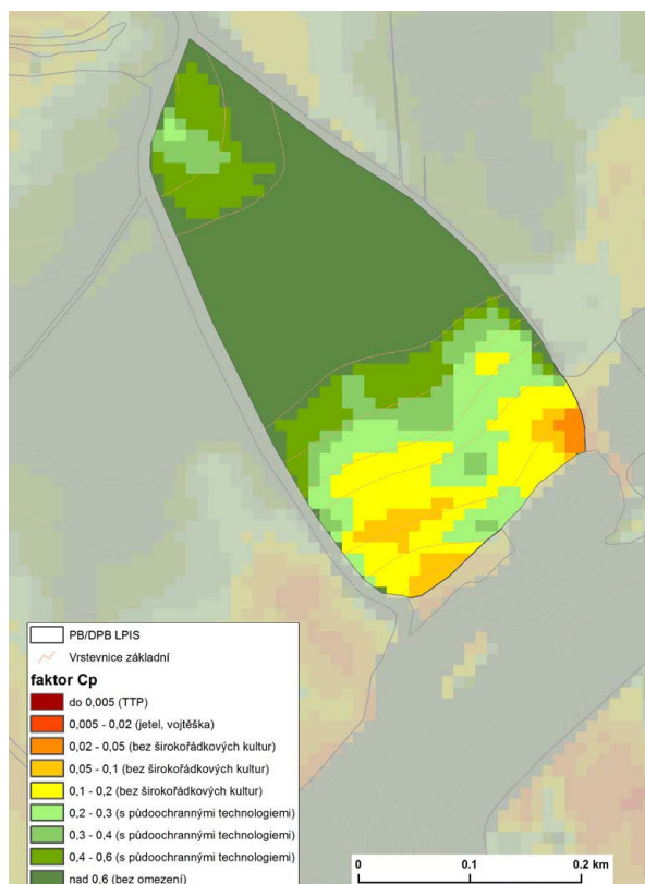
Obr. 2-16: Mapa Maximálních přípustných hodnot faktoru ochranného vlivu vegetace a protierozních opatření ( C_p \cdot P_p ) na DPB bez implementace krajinného prvku
