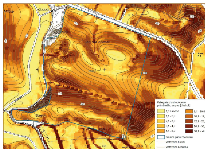
Obr. 3-8: Potenciální ohrožení dílu půdního bloku vodní erozí
