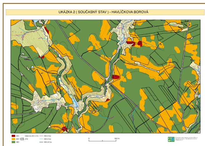
Obr. 2-3: Stávající vrstva erozní ohroženosti (EO) v rámci standardu DZES 5
