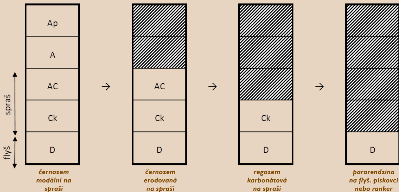
Obr. 3-17: Erodování původního půdního pokryvu a následný transport smytých půdních částic
