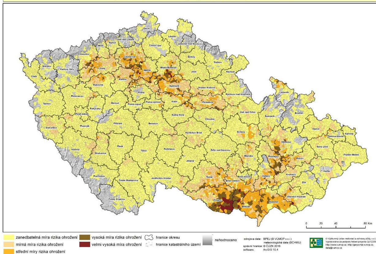
Obr. 6-15: Mapa rizika ohrožení orné půdy větrnou erozí podle katastrů
