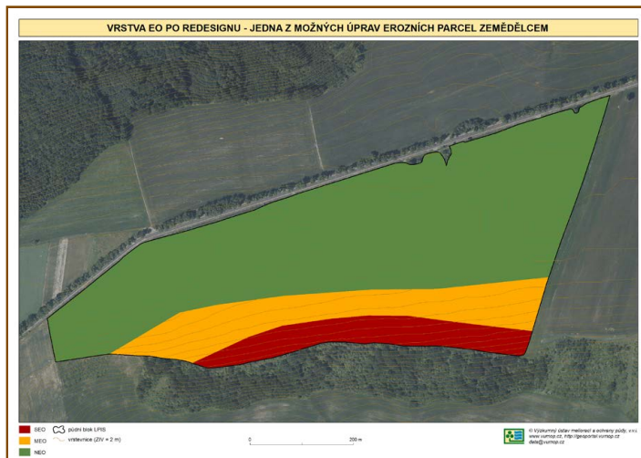
Obr. 2-8: Vrstva EO po redesignu – jedna z možných úprav erozních parcel zemědělce
