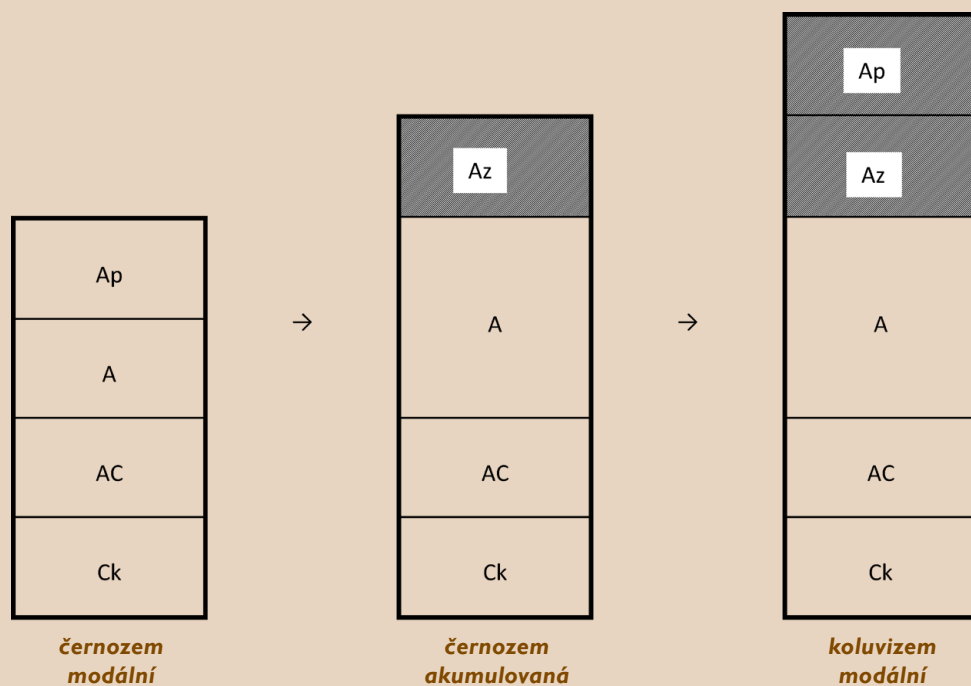
Obr. 3-18: Akumulace (ukládání) smyté půdy v depresních polohách (úpatí svahu)
