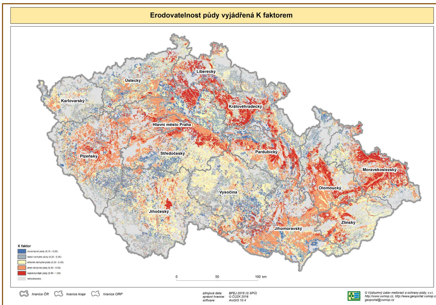
Obr. 2-20: Mapa faktoru erodovatelnosti půdy K
