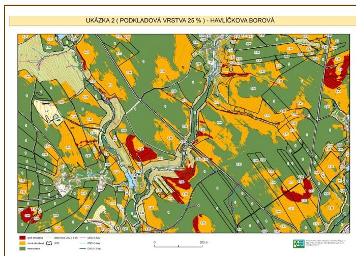
Obr. 2-4: Nová podkladová rastrová vrstva EO, převedená na 3 kategorie
