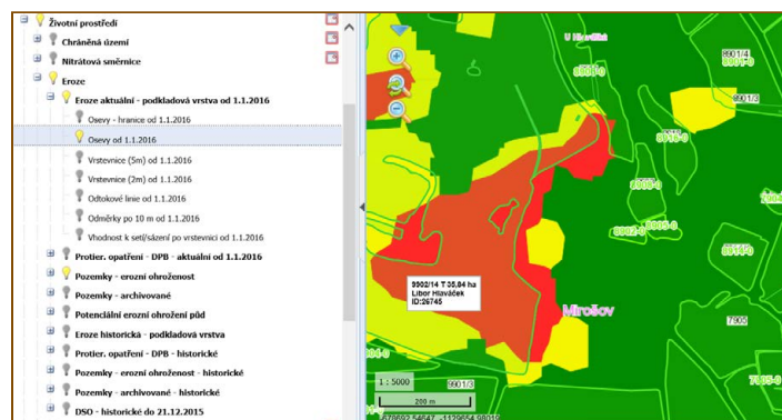
Obr. 2-26: Ukázka podkladové vrstvy erozní ohroženosti pro potřeby DZES 5 v LPIS
