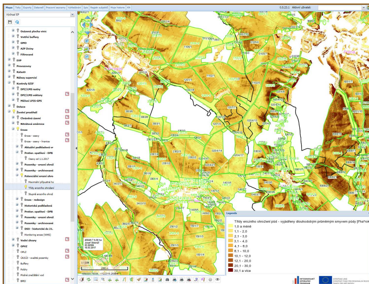
Obr. 7-4: Stupně erozní ohroženosti; zobrazení v LPIS
