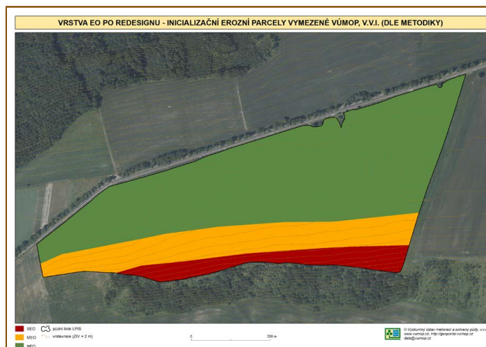
Obr. 2-7: Vrstva EO po redesignu – inicializační erozní parcely vymezené VÚMOP
