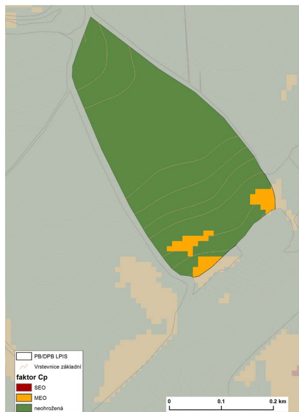
Obr. 2-17: Vrstva erozní ohroženosti v rámci Standardu DZES 5 na DPB bez implementace krajinného prvku
