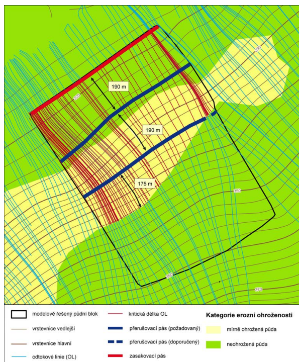
Obr. 2-39: Zasakovací pás Z3 založen na spodní hranici DPB doplněn o přerušovací pás ve vzdálenosti do 200 m od horní hrany zasakovacího pásu proti směru odtokových linií, druhý přerušovací pás doplněn ve vzdálenosti do 200 m od horní hrany prvního přerušovacího pásu proti směru odtokových linií, protože vzdálenost od horní hrany prvního přerušovacího pásu proti směru odtokových linií k horní hranici plochy MEO je větší než 200 m. Další přerušovací pás není nutné aplikovat, protože vzdálenost od horní hrany druhého přerušovacího pásu proti směru odtokových linií k horní hranici plochy MEO je menší než 200 m. (přerušované zobrazeno doporučené opatření)
