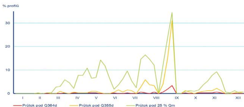
Graf 2.3.3 Změny průměrné vodnosti v hlásných profilech na území ČR v roce 2024
