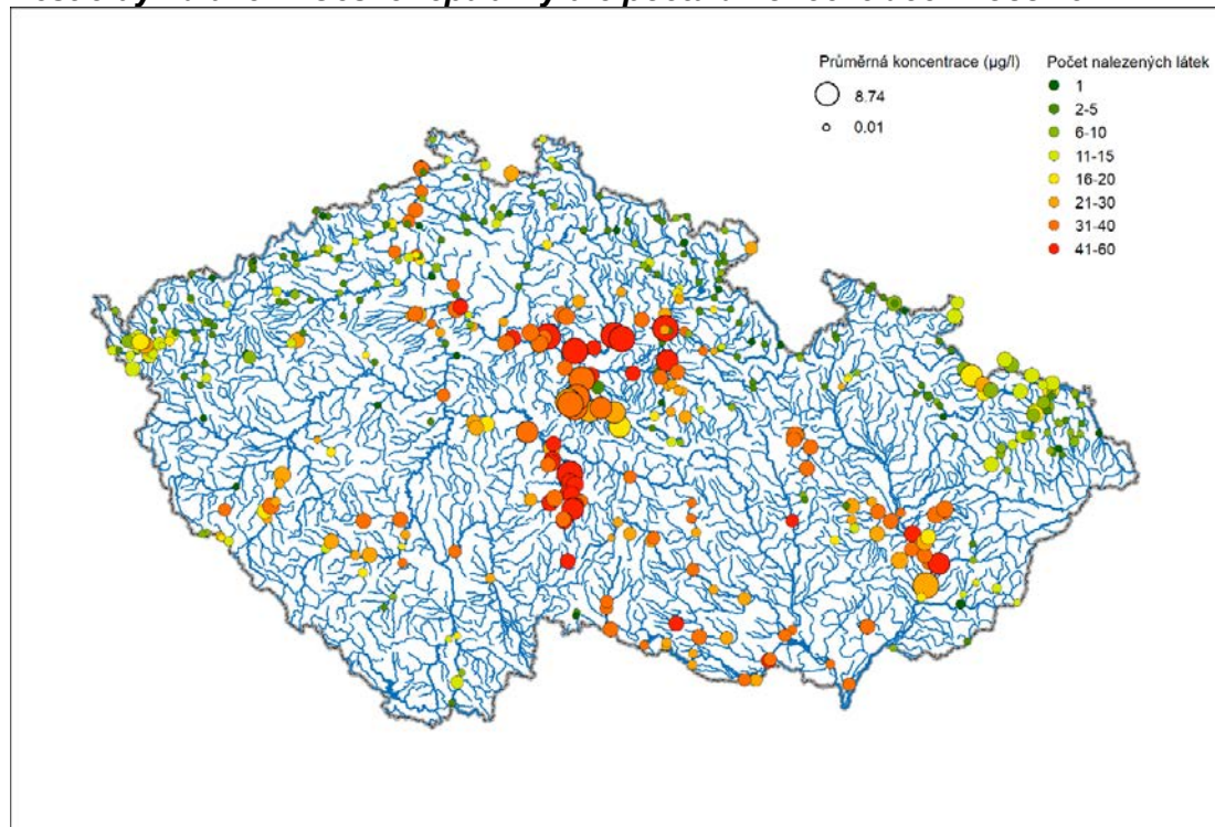
Obrázek 3.1.5 Pesticidy na území České republiky dle počtu a koncentrace v roce 2024
