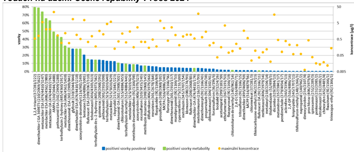
Graf 3.1.8 Frekvence výskytu povolených pesticidů a maximální dosažené koncentrace v povrchových vodách na území České republiky v roce 2024
